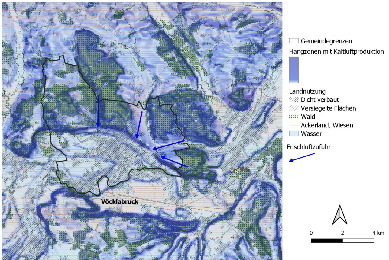
Abbildung 2: Klimafunktionskarte – Frischluft- und Kaltluftentstehungsgebiete für Vöcklabruck
