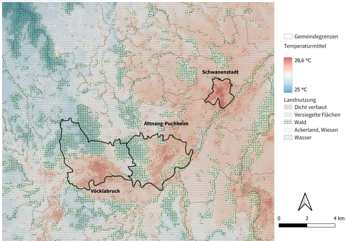
Abbildung 1: Überwärmungskarte für die Städte Vöcklabruck, Attnang-Puchheim und Schwanenstadt
