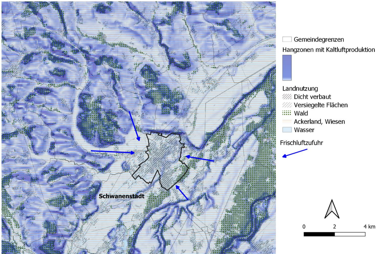
Abbildung 3: Klimafunktionskarte – Frischluft- und Kaltluftentstehungsgebiete für Schwanenstadt
