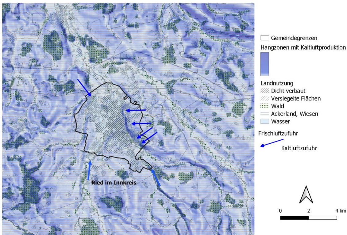
Abbildung 2: Klimafunktionskarte – Frischluft- und Kaltluftentstehungsgebiete für Ried
