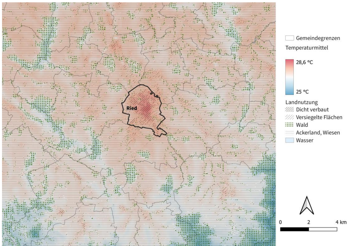
Abbildung 1: Überwärmungskarte für Ried
